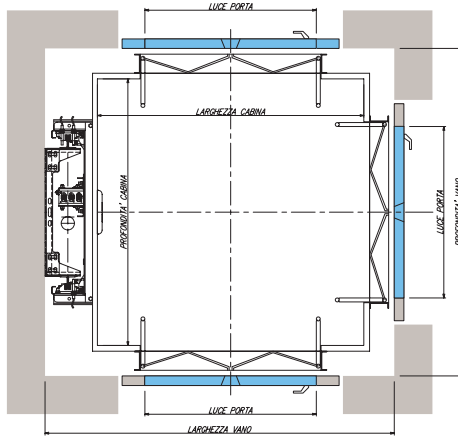
Tre accessi Three entrances
